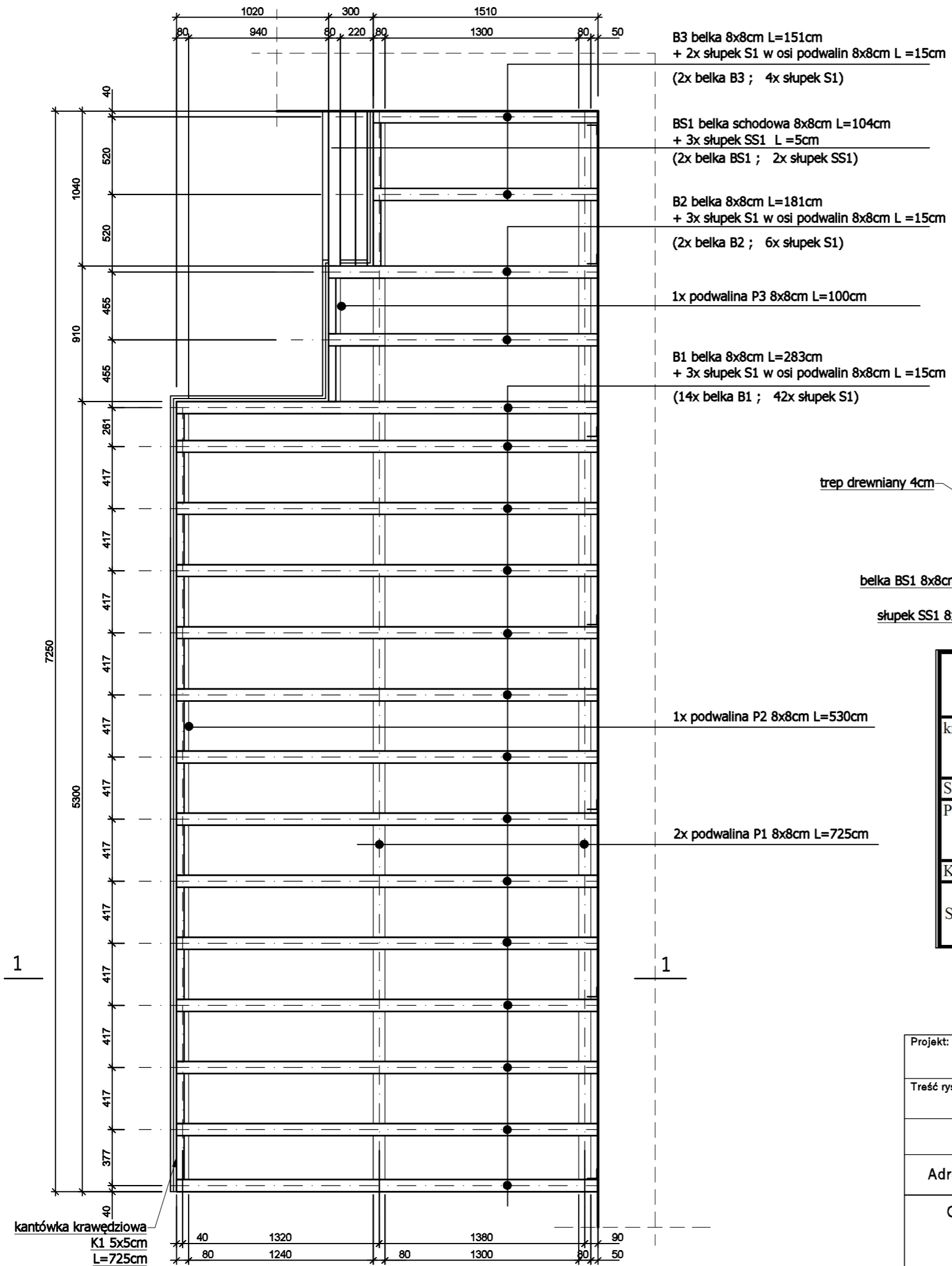
konstrukcja schodka
