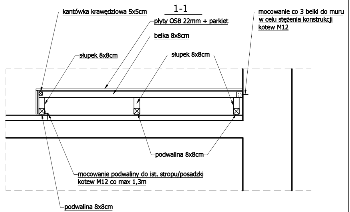
konstrukcja schodka
