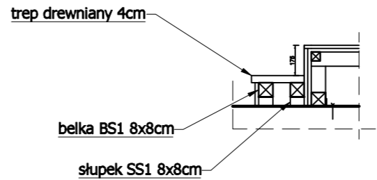
konstrukcja schodka
